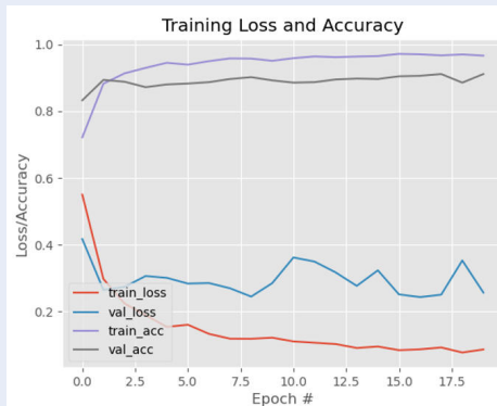
Hình 7: Biểu đồ Training loss và Training accuracy
