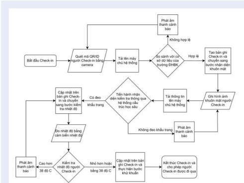
Hình 3: Lưu đồ xử lý thông tin để kết luận các trường hợp người Check-in được phép hay không được phép đi qua
