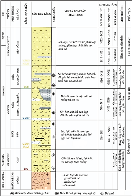
Hình 2: Cột địa tầng tổng hợp bồn trũng Nam Côn Sơn. 8
